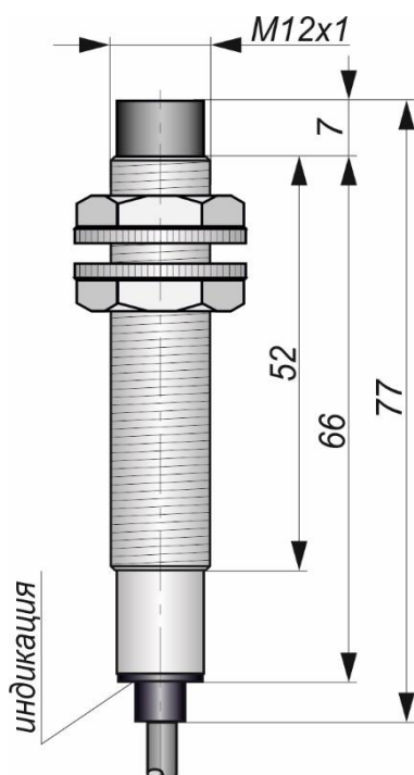
Габаритный чертеж
